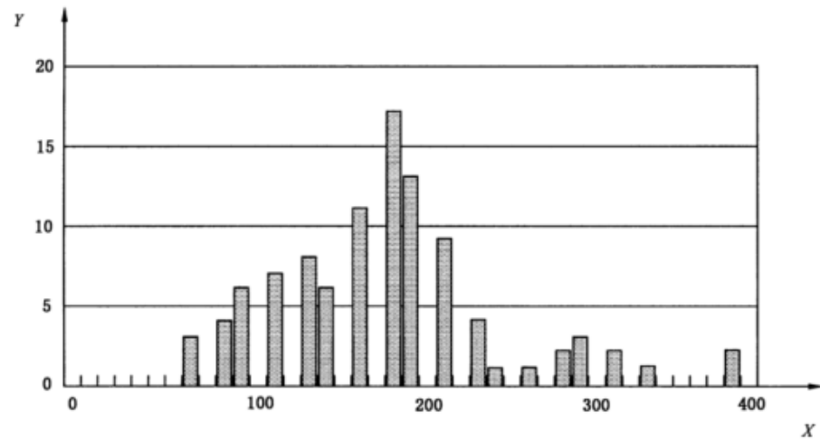
图 A.1 使用搅拌器研磨并筛分后的 PLA 粉末的粒径分布
